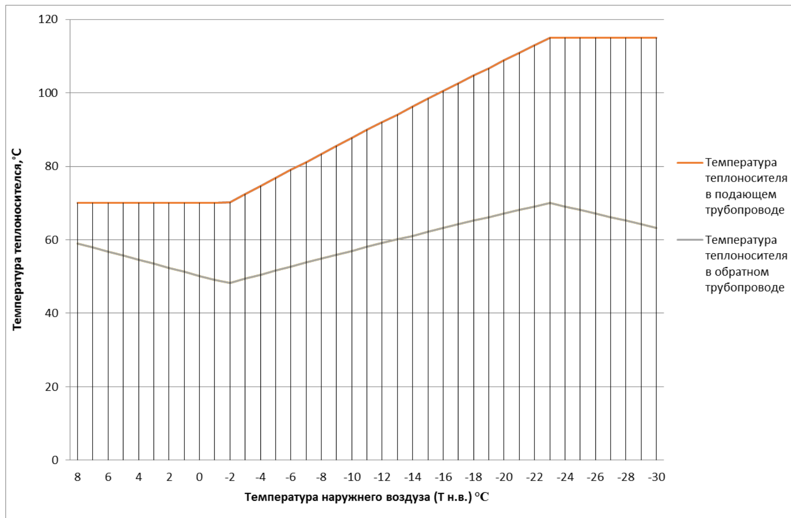
Рис. 1. Температурный график 115/70 °С работы источника тепловой энергии ГТЭЦ, котельная «Журавлики»
