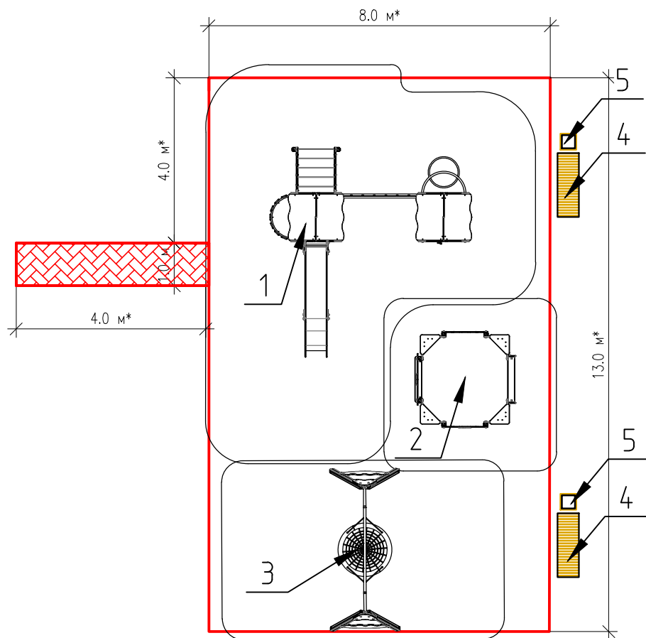
Детская площадка (эскизный план)
